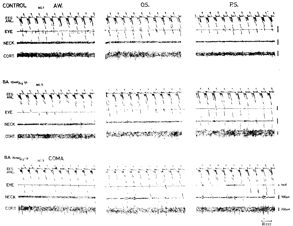
圖一 各種濃度之 B. A. 對老鼠睡眠型式之影響 CONTROL：(對照組) AW.：覺醒期 O. S.：正常睡眠期 P. S.：反常睡眠 EEG ANAL：腦波分析積分植 (10 秒間) 由前面後各為 2-4, 4-8, 8-13, 13-20, 20-30 Hz EYE：眼球之運動 NECK：頸肌肌電圖 CORT：運動感覺區腦波 (以下各圖之略稱皆與上同) B. A.：Butyric acid COMA：昏睡期 校正 1 mV, 50 μV 及 200 μV 及 10 sec 各行共通使用
