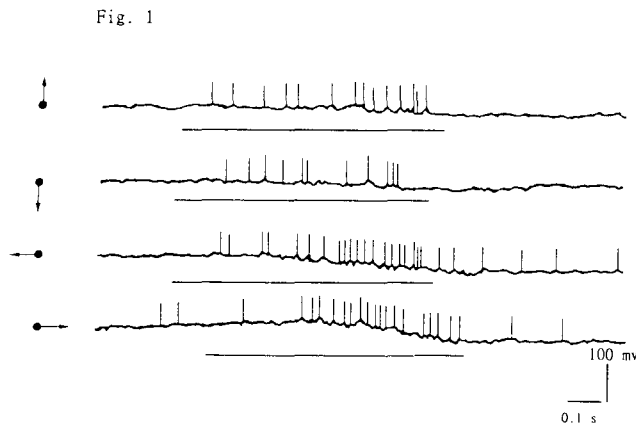
圖一、lobula 內沒有方向性神經原胞內記錄的一例箭頭表示電腦輝點從中心移動的方向。每條記錄下之橫線表示輝點出現後移動所需之時間。
