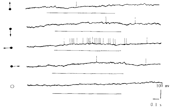
圖三、lobula 內單方向性神經原胞內記錄的一例，圖中最下「○」者表示輝點出現，但未移動時的胞內記錄。
