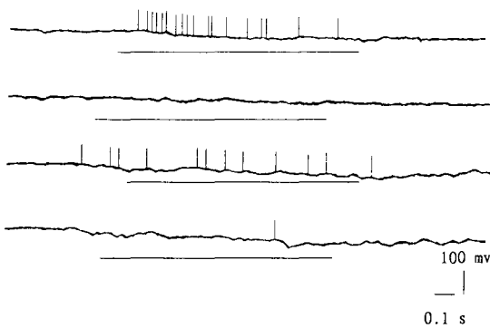
圖二、lobula 內二方向性神經原胞內記錄的一例。
